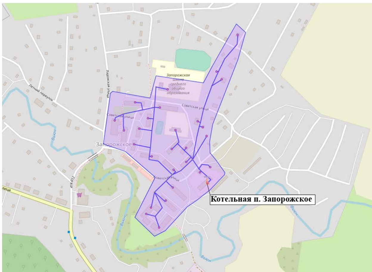
Рисунок 1 Зона действия котельной п. Запорожское
