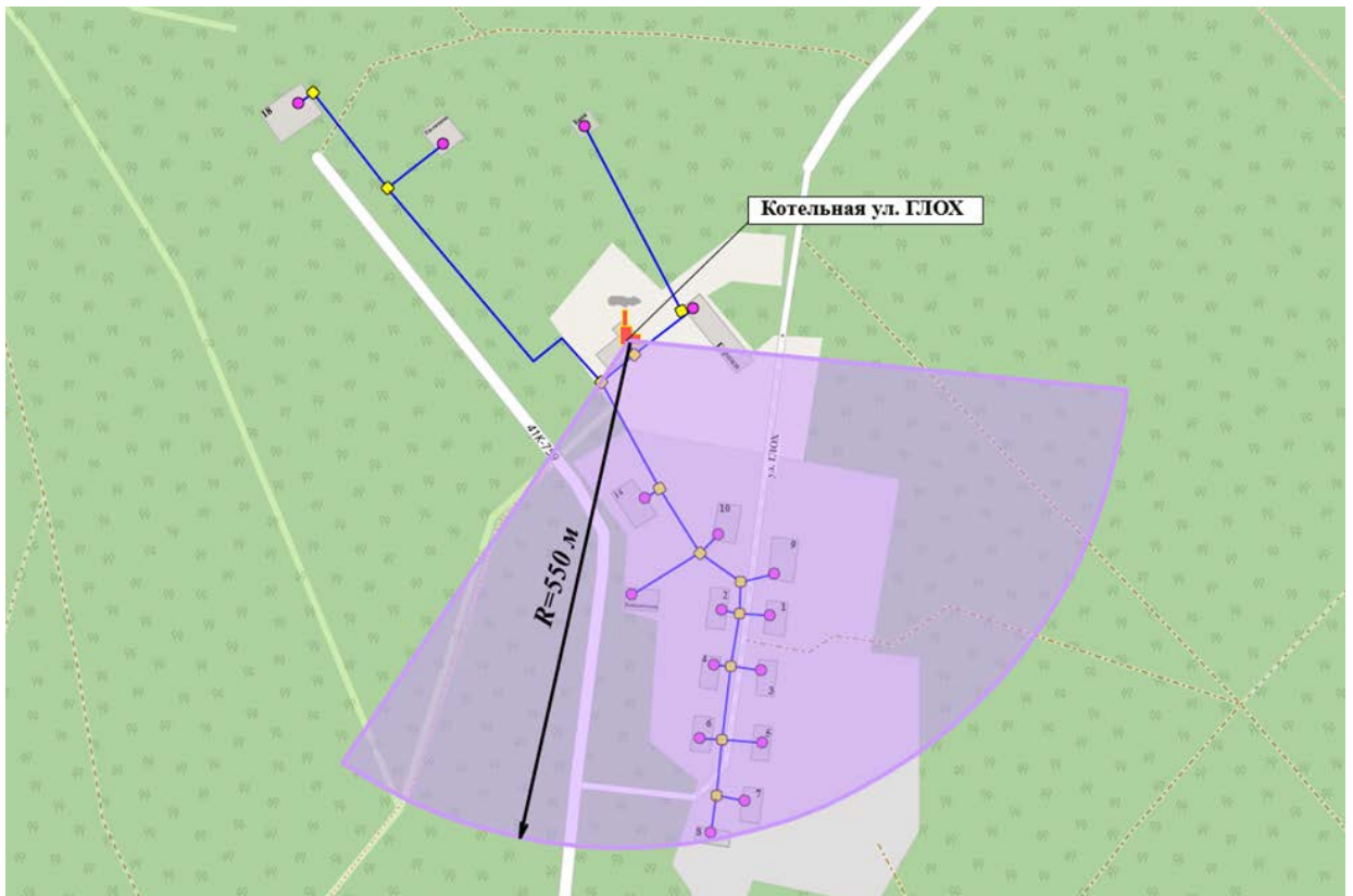
Рисунок 4 Тепловая зона и радиус эффективного теплоснабжения котельной ГЛОХ
