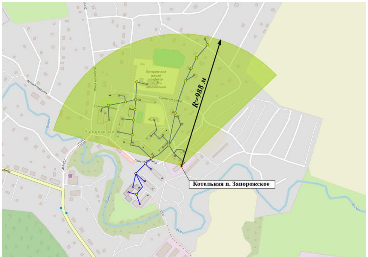
Рисунок 3 Тепловая зона и радиус эффективного теплоснабжения котельной п. Запорожское
