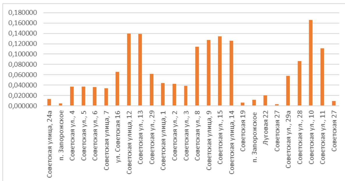
Рисунок 42 Средний суммарный недоотпуск теплоты потребителям от котельной п. Запорожское
