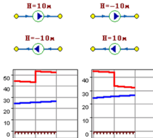
Рисунок 29 Пьезометрические графики
