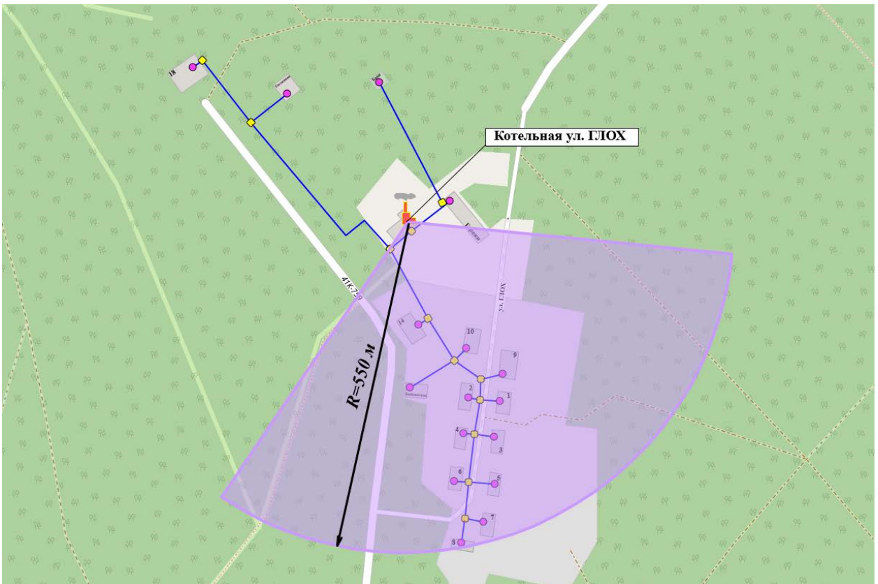
Рисунок 39 Тепловая зона и радиус эффективного теплоснабжения котельной ГЛОХ
