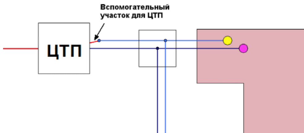
Рисунок 19 Подключение трубопровода ГВС
