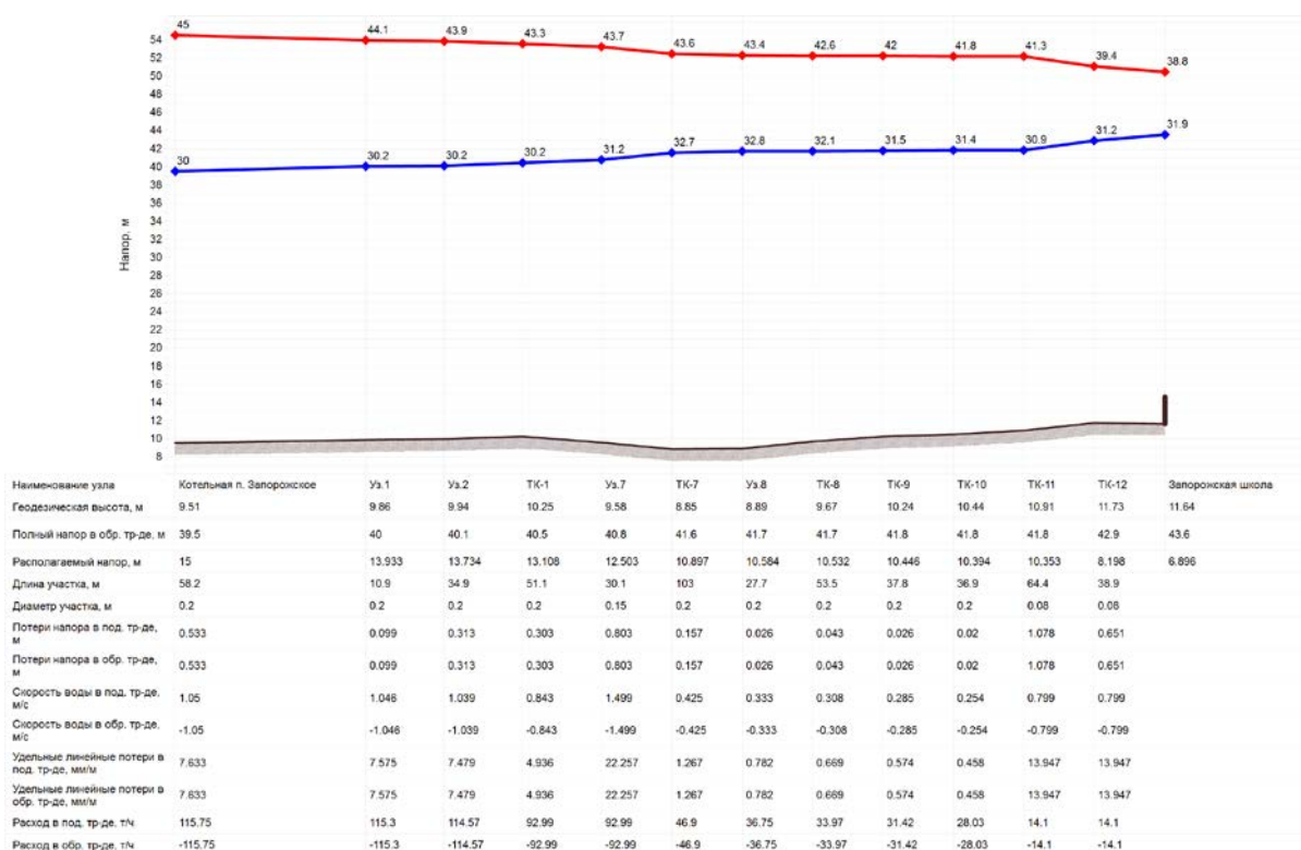
Рисунок 37 Пример пьезометрического графика
