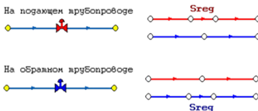
Рисунок 31 Дросселирующие устройства
