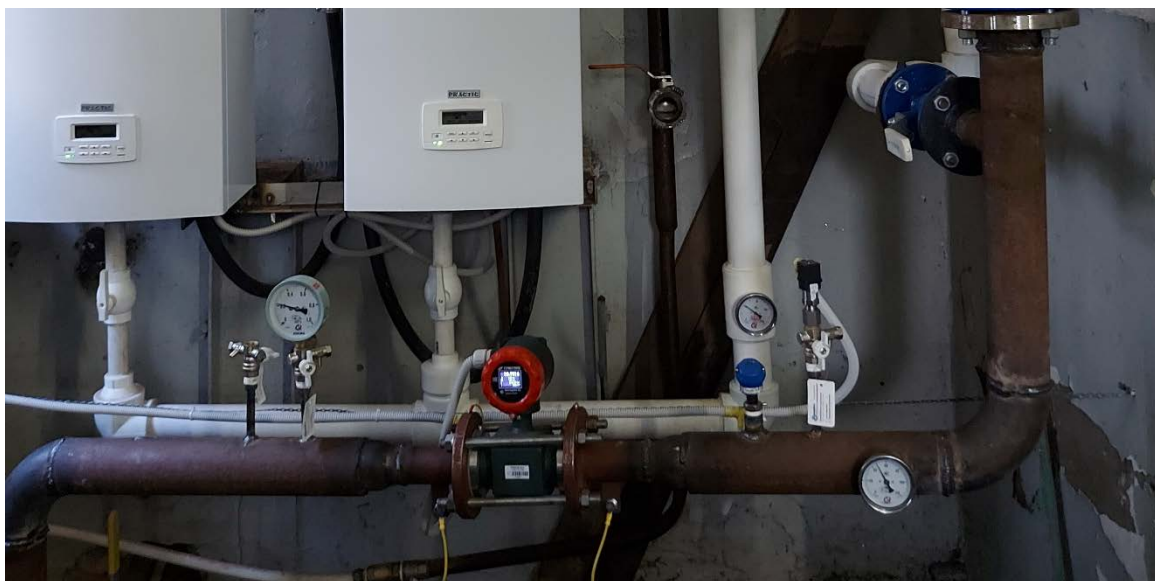
Рисунок 7 Внешний вид узла учета подающего трубопровода тепловой энергии, установленного на котельной ГЛОХ
