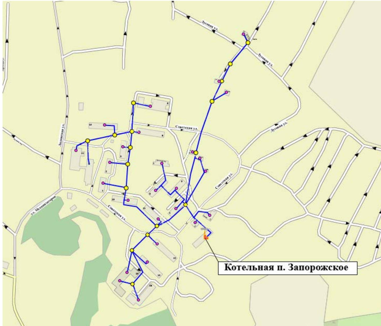
Рисунок 9 Схема тепловых сетей котельной п. Запорожское
