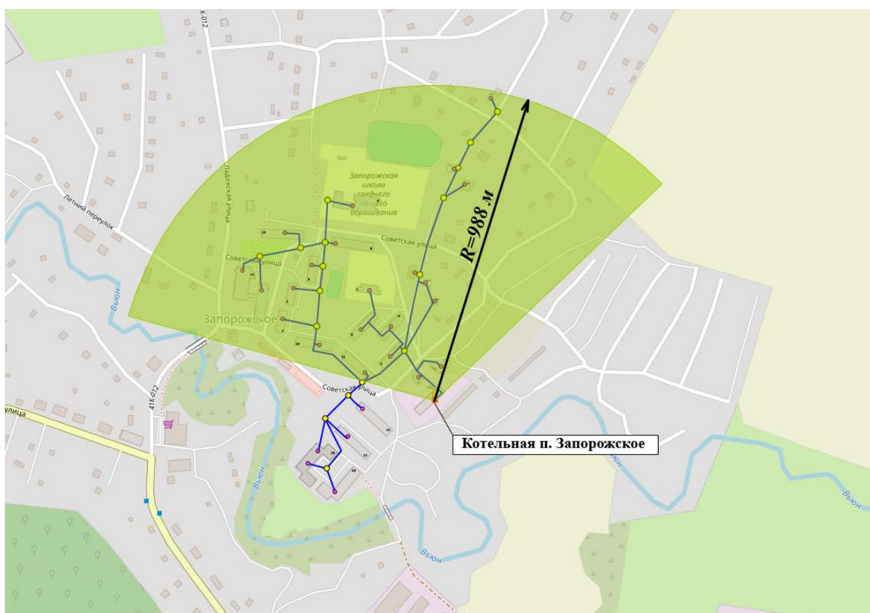
Рисунок 38 Тепловая зона и радиус эффективного теплоснабжения котельной п. Запорожское
