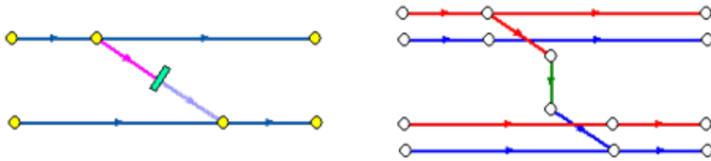
Рисунок 27 Соединение между подающим трубопроводом одного участка и обратным трубопроводом другого участка
